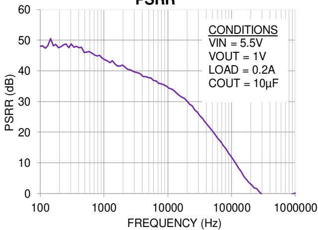
PSRR
